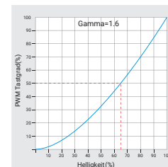
Logarithmische Dimmkurve
